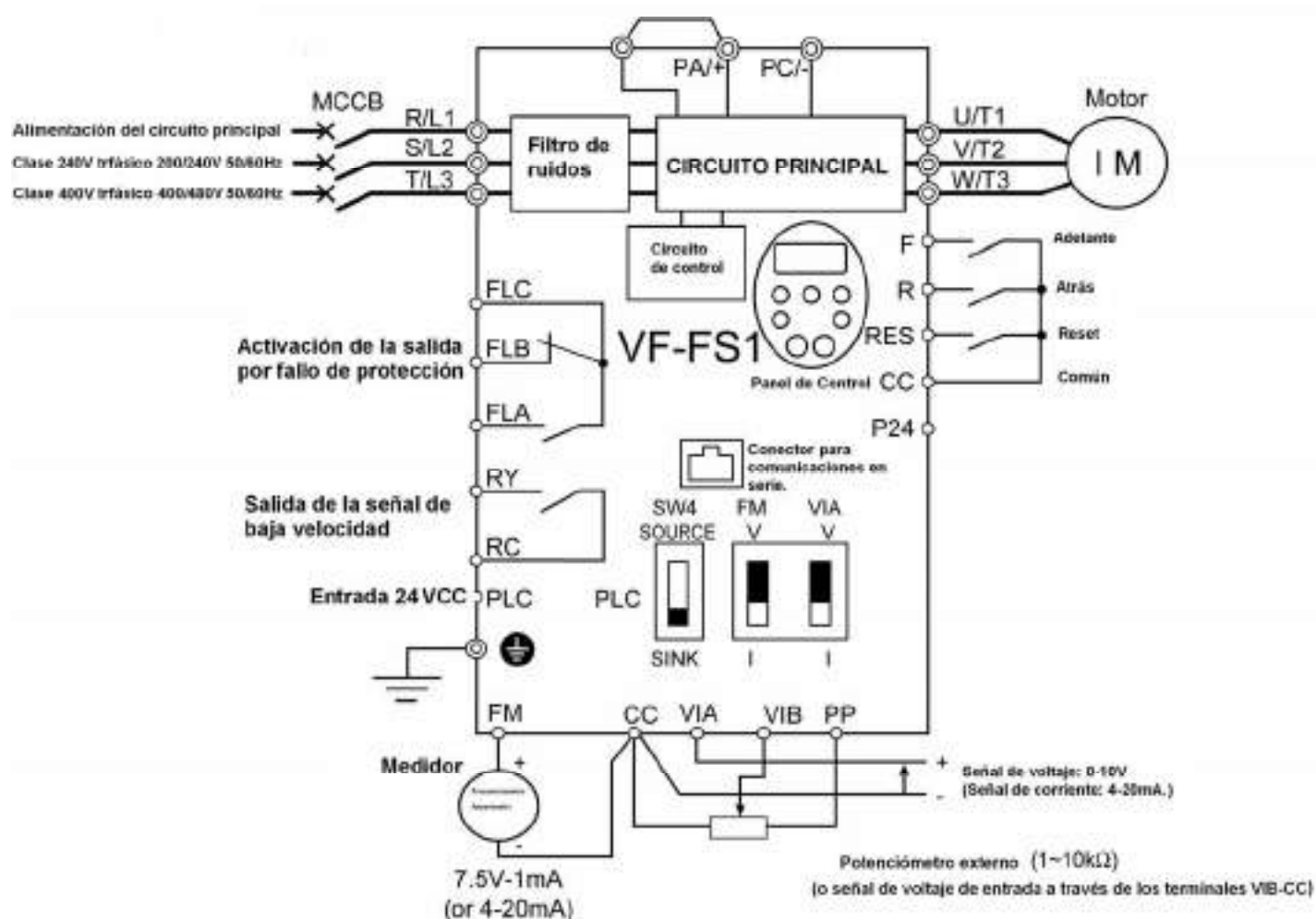
Diagrama de conexión estándar -SINK (Negativa) (común:CC)
